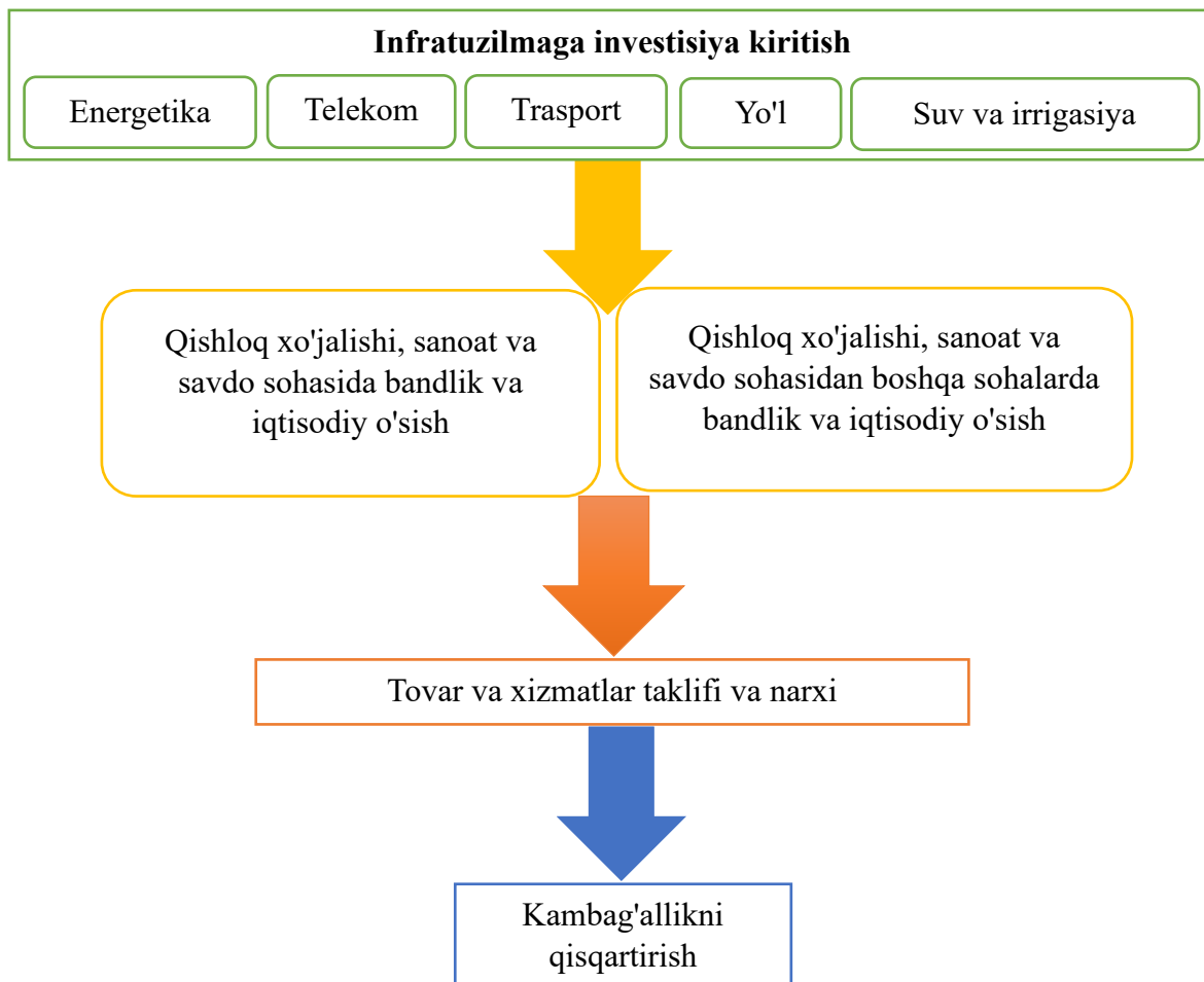
1-rasm. Kambag'allik va infratuzilma investisiyalari o'rtasidagi mantiqiy bog'liqlikni ko'rsatuvchi model 45
